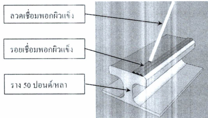
ภาพที่ 2 การจำลองลักษณะกระบวนการเชื่อมพอกผิวแข็งรางรถไฟ
