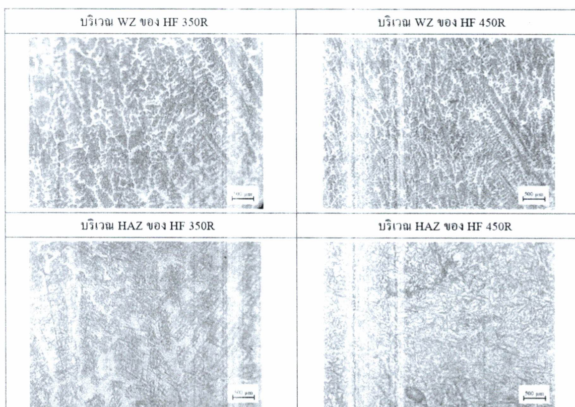
ภาพที่ 6 โครงสร้างจุลภาคจากการเชื่อมพอกผิวเชิงรางรถไฟ บริเวณรอยเชื่อม (WZ) บริเวณที่ได้รับอิทธิพลจากความร้อน (HAZ) บริเวณเนื้อโลหะเดิม (BM)
