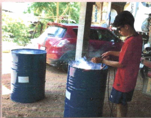
ภาพที่ 3 ขั้นตอนการสร้างเครื่องกรองน้ำ และเตาเผาถ่านอุณหภูมิสูงแบบไร้ควัน
