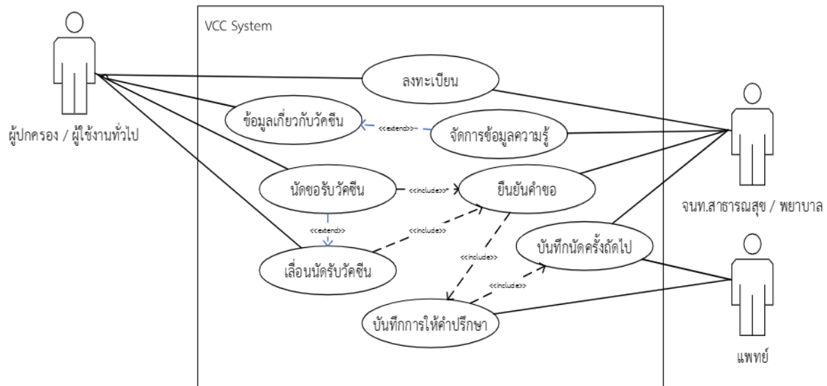
รูปที่ 2 Use Case Diagram
