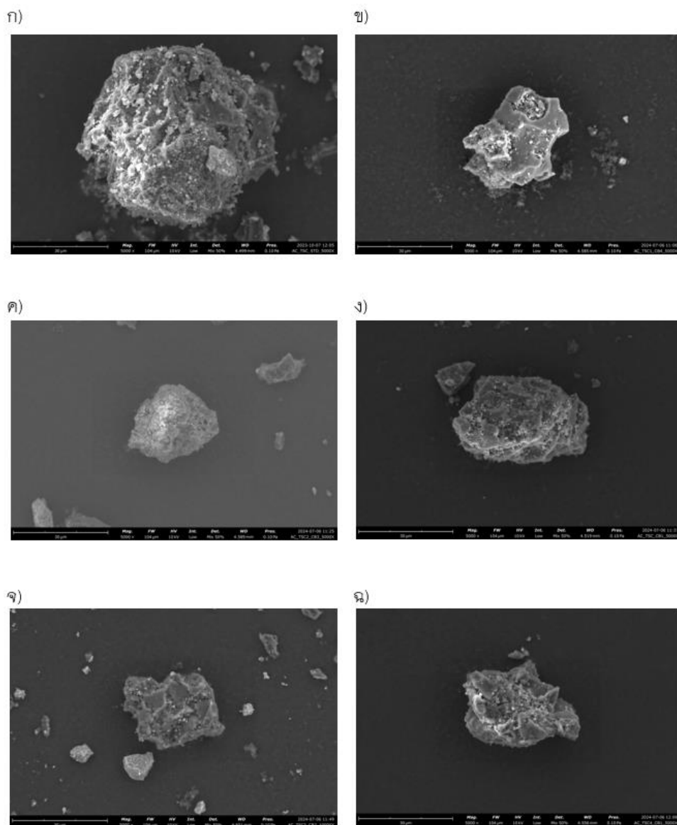
ภาพที่ 2 ภาพถ่ายพื้นผิวของ ก) ถ่านกัมมันต์จากเมลล็ดมะขามและถ่านกัมมันต์จากเมลล็ดมะขามที่ผสมกับคาร์บอนแบล็คในสัดส่วน ข) 1.00 : 4.00 ค) 1.00 : 1.50 ง) 1.00 : 1.00 จ) 1.00 : 0.67 และ ฉ) 1.00 : 0.25
