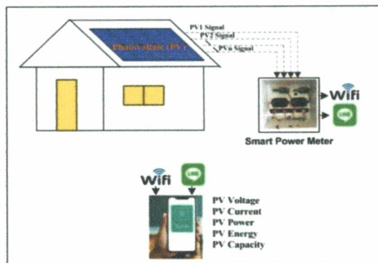
ภาพที่ 1 รูปแบบการทำงานเครื่องวัดกำลังไฟฟ้าอัจฉริยะสำหรับการติดตามสมรรถนะ แผงผลิตไฟฟ้าพลังงานแสงอาทิตย์
