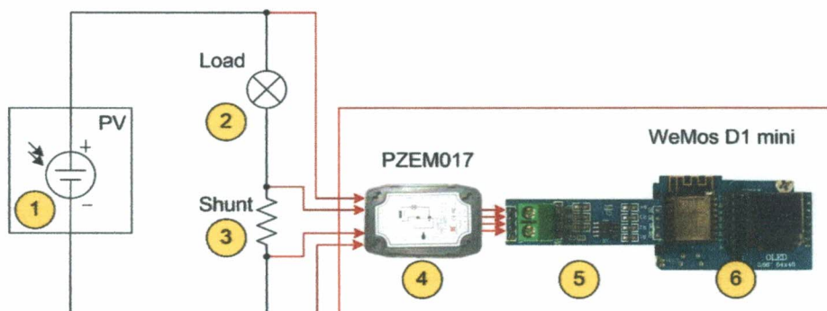
ภาพที่ 2 อุปกรณ์หลักและการเชื่อมต่ออุปกรณ์เครื่องวัดกำลังไฟฟ้า
