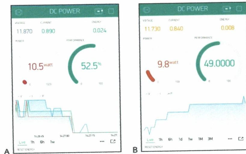
ภาพที่ 6 หน้าจอการแสดงผลบนสมาร์ตโฟนด้วยแอปพลิเคชันบลิงค์ (A) เครื่องวัดกำลังไฟฟ้าชุดที่ 1 และ (B) เครื่องวัดกำลังไฟฟ้าชุดที่ 2
