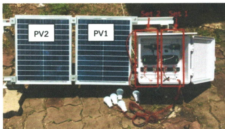
ภาพที่ 3 การติดตั้งเครื่องวัดกำลังไฟฟ้ากับชุด PV
