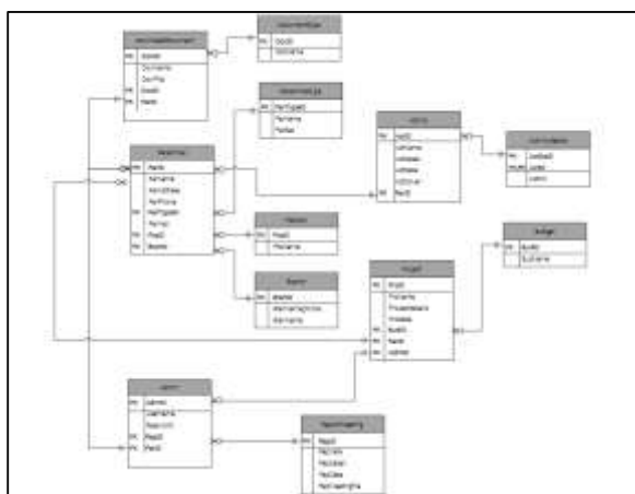
ภาพที่ 2 แบบจำลองอี-อาร์ไดอะแกรม ออกแบบฐานข้อมูล
