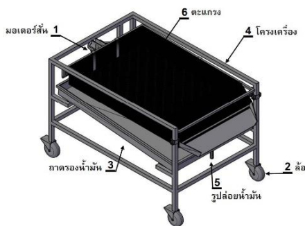
รูปที่ 4 แบบเครื่องสับตักน้ำมัน
