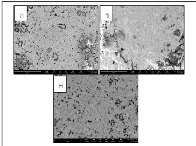
ภาพประกอบ 2 ภาพถ่ายพื้นผิวของอนุภาคของฟิล์ม \text{TiO}_2 ที่เจือด้วย \text{Al}_2\text{O}_3 เฝ้านิกส์สารที่อุณหภูมิ ก) 900 °C ข) 950 °C และ ค) 1000 °C
