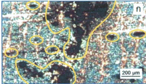
ก. ลวดเชื่อมชนิด H450R
