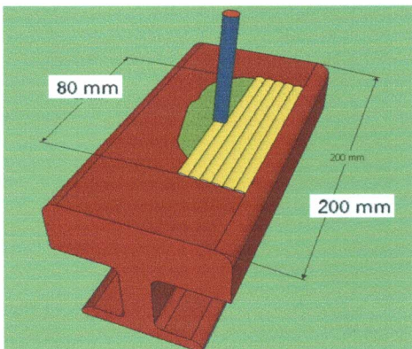
รูปที่ 2 แบบจำลองการเชื่อมพอกแข็งบนเหล็กกล้ารางรถไฟ
