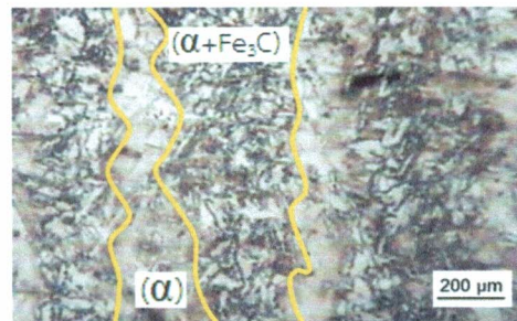
รูปที่ 5 การตรวจสอบโครงสร้างจุลภาคบริเวณเนื้อโลหะเดิม (BM)
