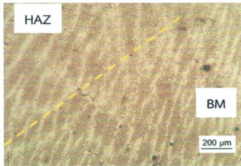
รูปที่ 8 การตรวจสอบโครงสร้างจุลภาคบริเวณ ที่ได้รับอิทธิพลจากความร้อน (HAZ) กับบริเวณรอยเชื่อม (WZ) ของลวดเชื่อม H450R
