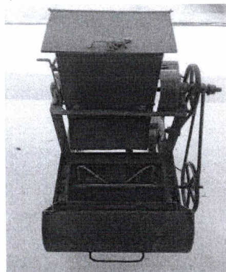
(ข) ชุดบดถ่านและผสมถ่านดัดแปลงจากชุดบดน้ำแข็ง
