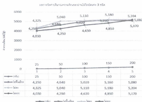
รูปที่ 8 ผลการวัดค่าปริมาณความร้อนจากถ่านไม้ไผ่อัดแท่งทั้ง 3 ชนิด
