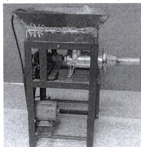
(ค) ชุดอัดถ่านดัดแปลงจากเครื่องบดหมู
