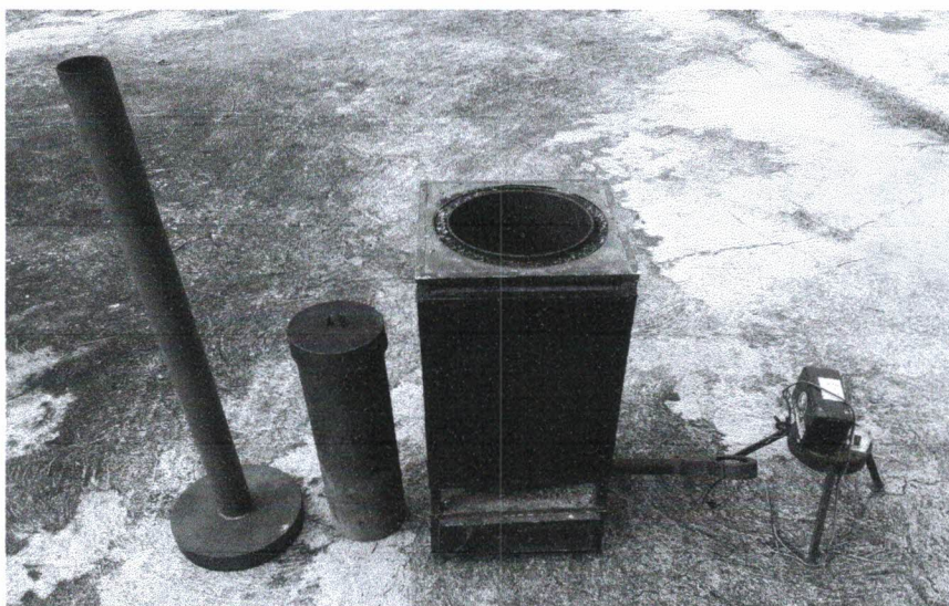
ภาพที่ 2 ลักษณะของเตาประดิษฐ์สำหรับการเผาถ่านจากเศษกะลามะคาเดเมียที่ใช้ในการศึกษา
