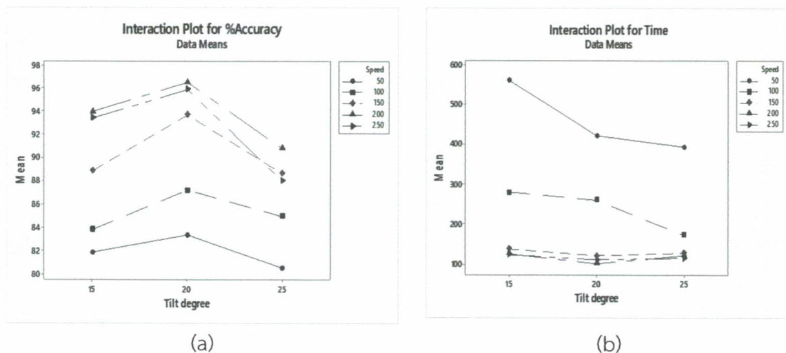
ภาพที่ 7 กราฟการวิเคราะห์ปัจจัยที่ส่งผลต่อเปอร์เซ็นต์ความแม่นยำและเวลาในการคัดขนาด (a) Interaction Plot ที่ส่งผลต่อความแม่นยำ และ (b) Interaction Plot ที่ส่งผลต่อเวลา
