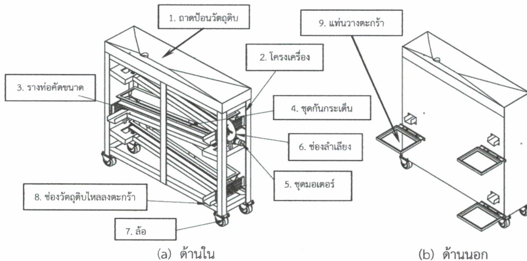
ภาพที่ 2 แบบงานเครื่องคัดขนาดกะลาแมคคาเดเมียแบบชั้นรางท่อ (a) ด้านใน และ (b) ด้านนอก
