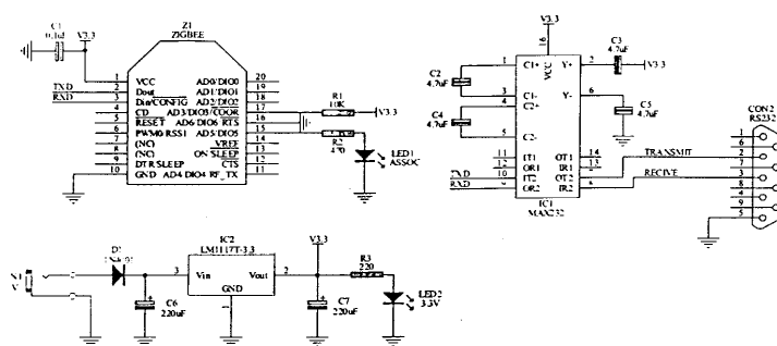
รูปที่ 3.3 วงจรสมบรูณ์ภาครับ
